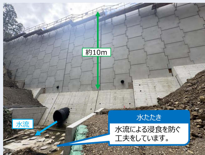
擁壁の整備状況（令和8年8月12日撮影）
